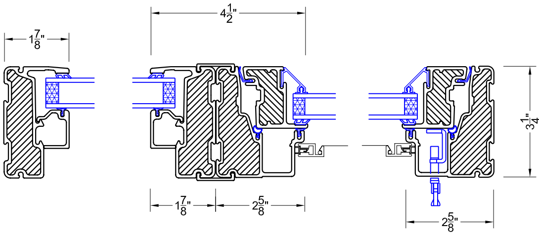
JAMB DETAIL
