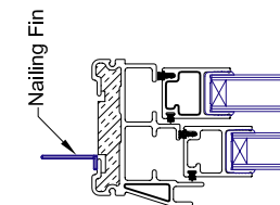
400 DHT Frame Jamb
