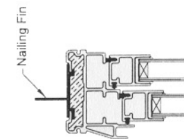
400 DHT Frame Jamb
