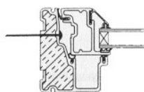
Casement Frame Jamb
