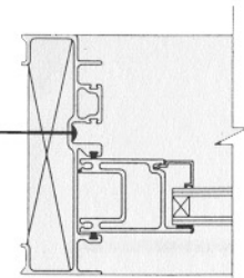
Patio Door Frame Jamb
