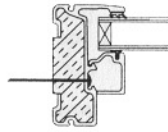
Fixed Frame Jamb
